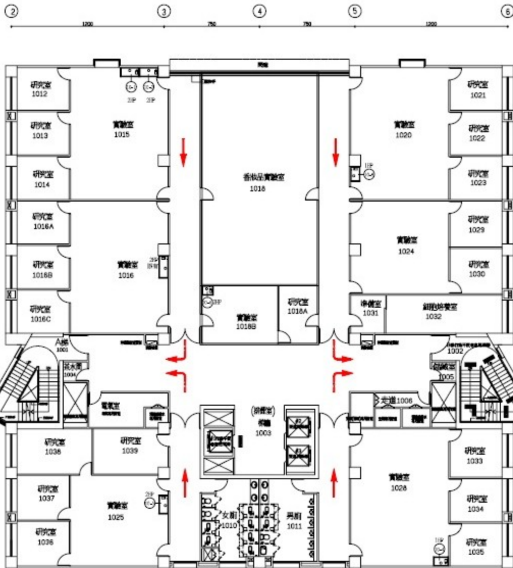
教學大樓 10F平面圖(FT) 逃生路線
