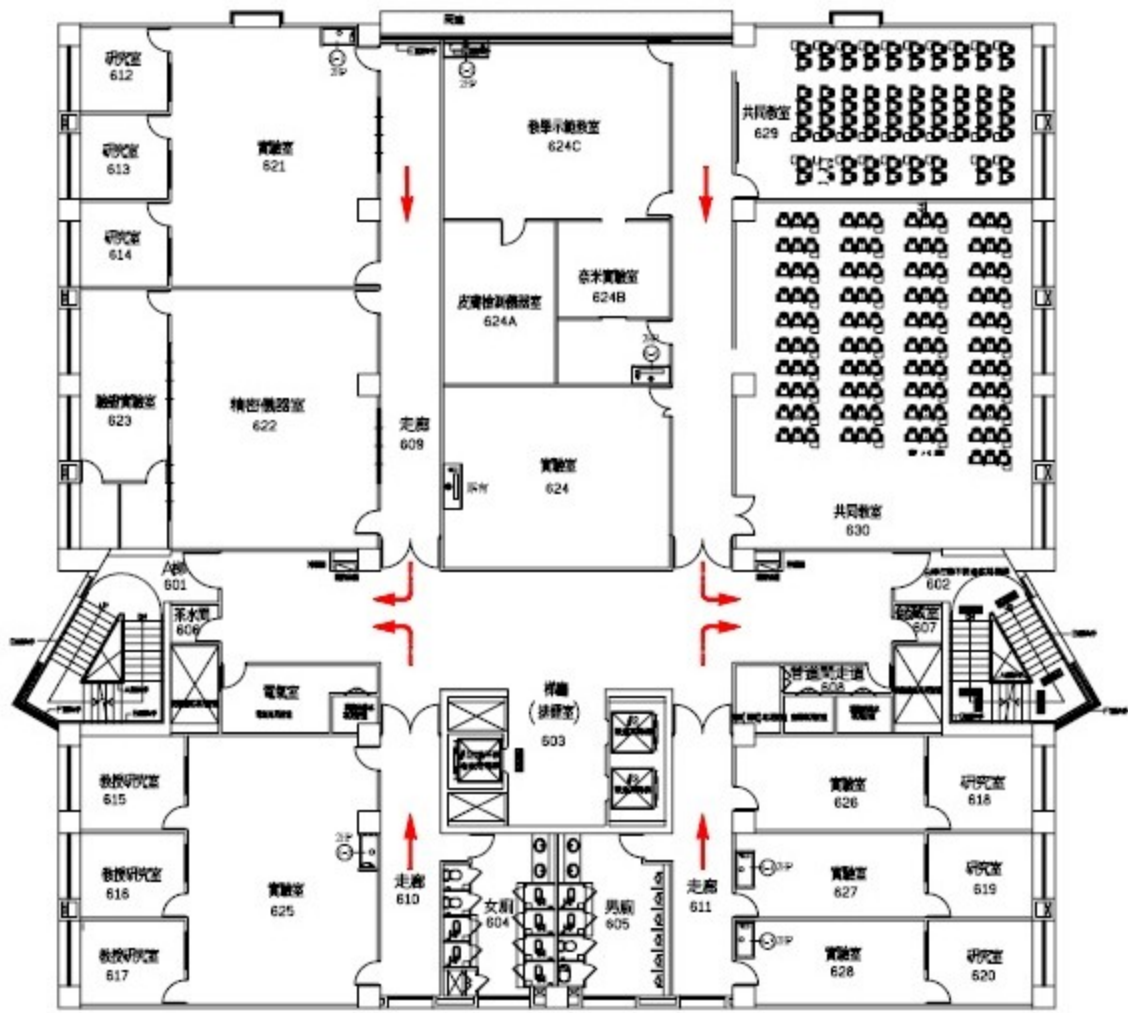
教學大樓 6F 平面圖(FT) 逃生路線
