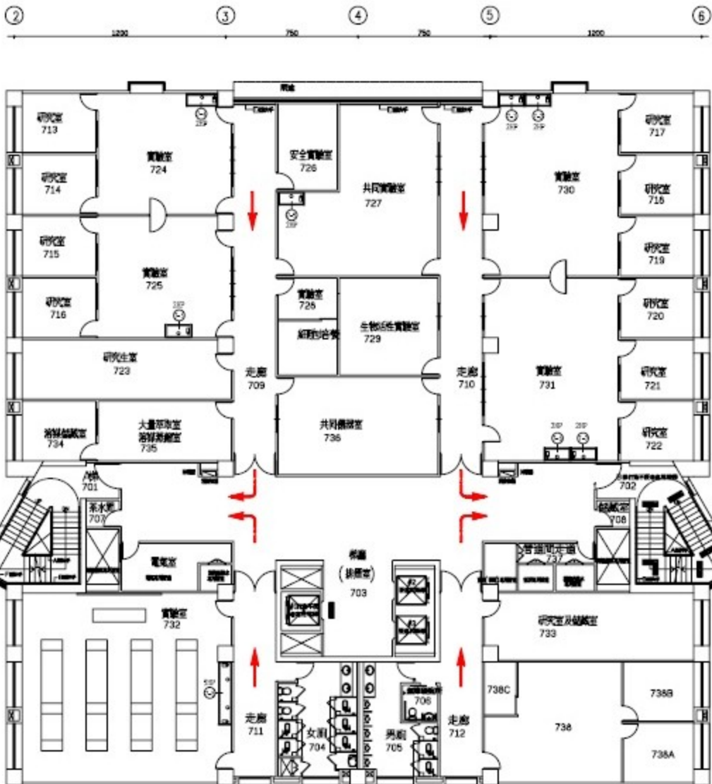
教學大樓 7F 平面圖(FT) 逃生路線
